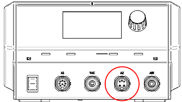
Abbildung / Figure 2: A2 Anschluss / socket i-CON VARIO 2
